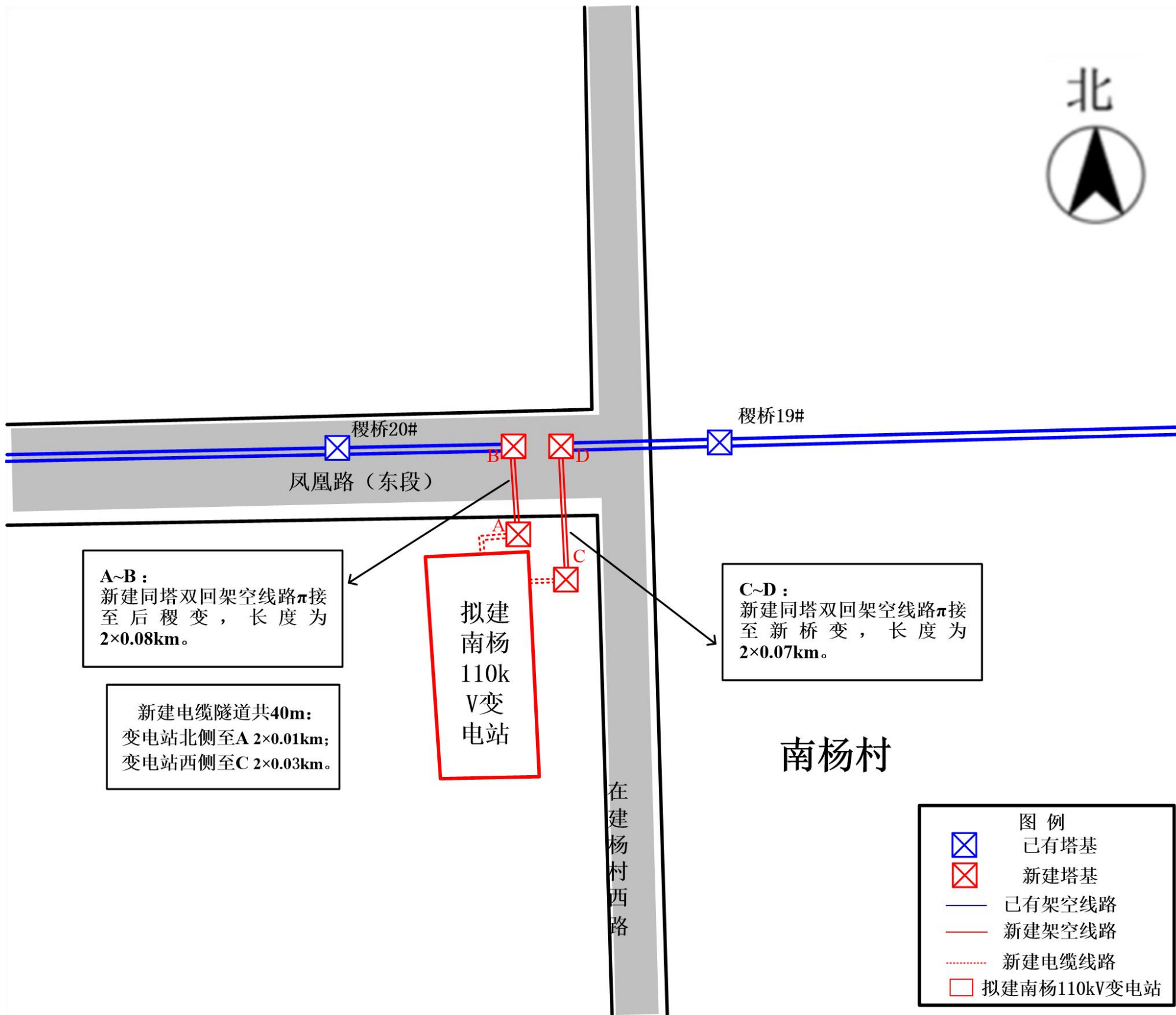
图 2-5 本工程输电线路走径示意图
