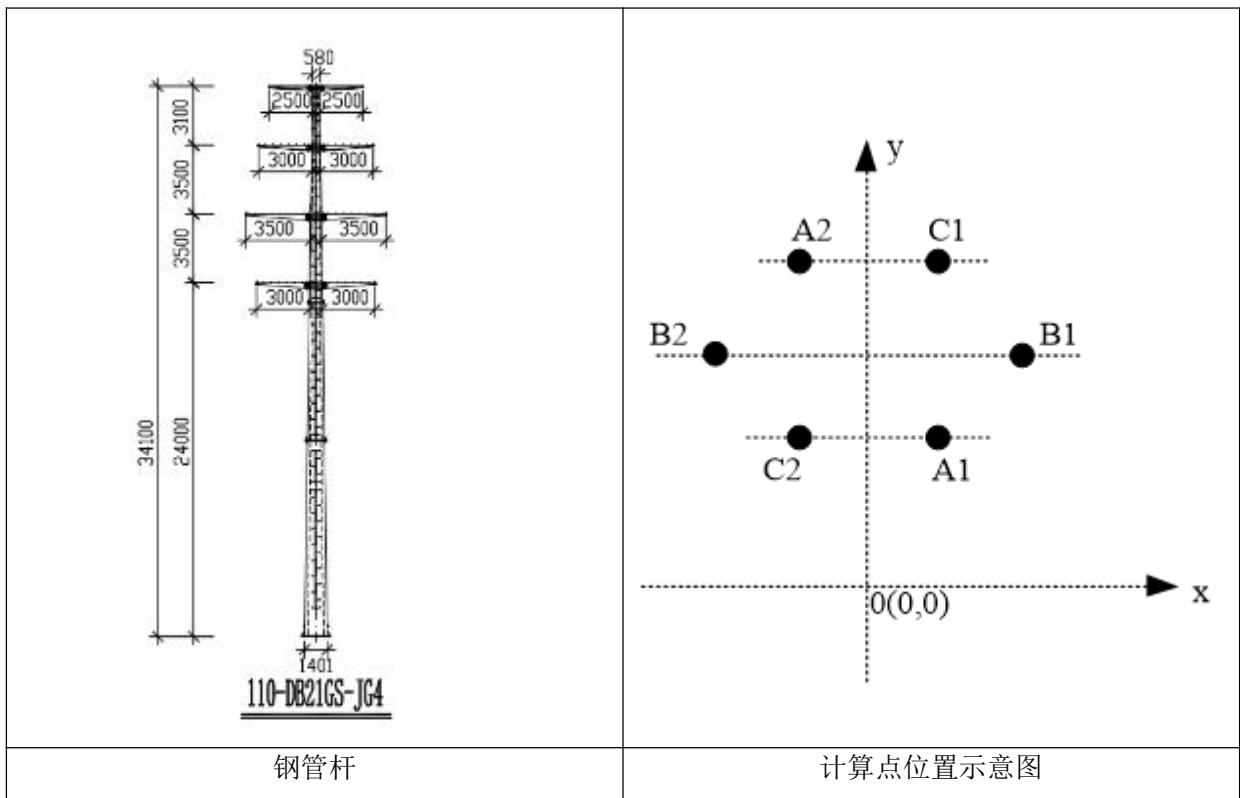
图 2 预测塔型图和计算点位置示意图
