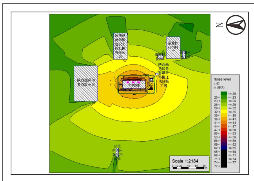
图 4-7 拟建南杨 110kV 变电站声环境预测等值线示意图
