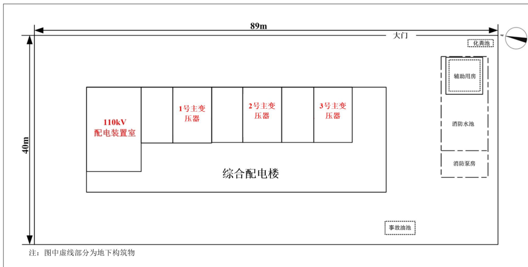
图 2-3 南杨 110kV 变电站平面布置示意图
