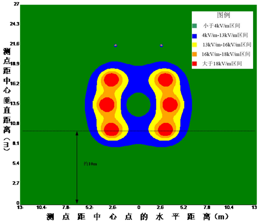
图5 110-DC31D-ZM2 架空线空间截面电场强度分布图
