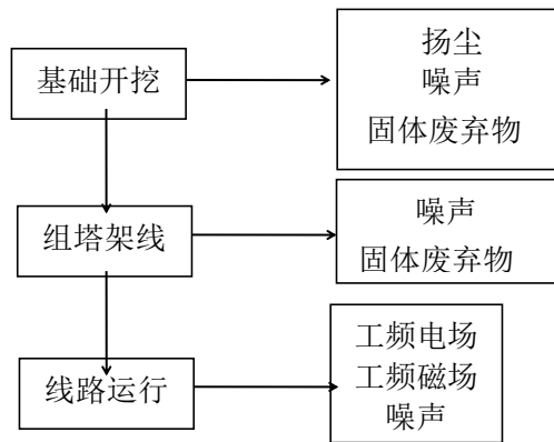
图 4-2 架空线路施工期工艺流程及产污环节示意图
