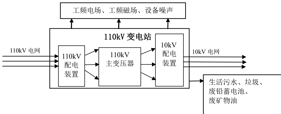
图 4-6 本项目变电站运行期产污环节示意图
