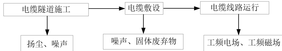
图 4-1 电缆线路施工期工艺流程及产污环节示意图
